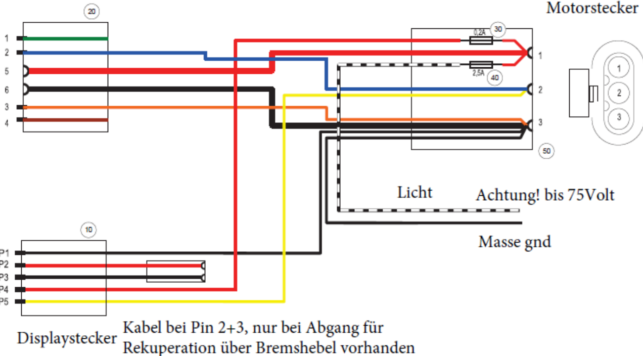
Motorstecker
